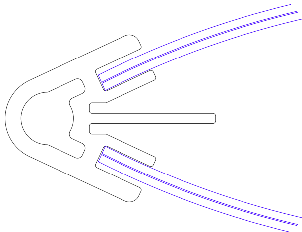
Pylonprofil doppelseitig Scheibeneinschub
