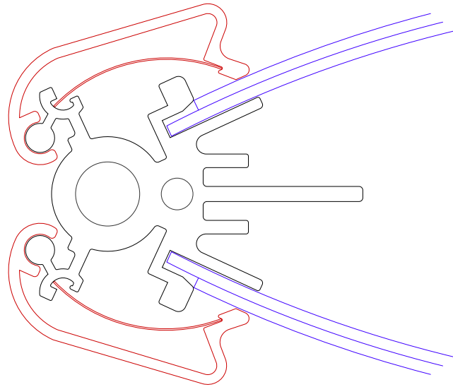
Pylonprofil doppelseitig Klappe 32 mm
