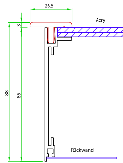
Steckrahmen mit 26,5 mm Abdecksteckleiste
