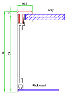
Steckrahmen mit 16,5 mm Stecksteckleiste
